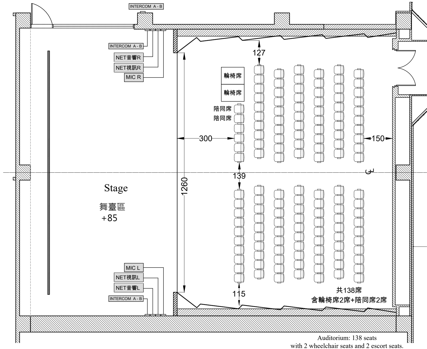
圖 (三) 小舞台(3201)_座位圖及音響視訊配置圖 (單位：公分) Figure(3) Small Stage(3201)_Auditorium Plan and Audio & Video Plan (Unit: cm)
